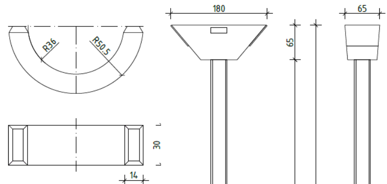
Koppelring
